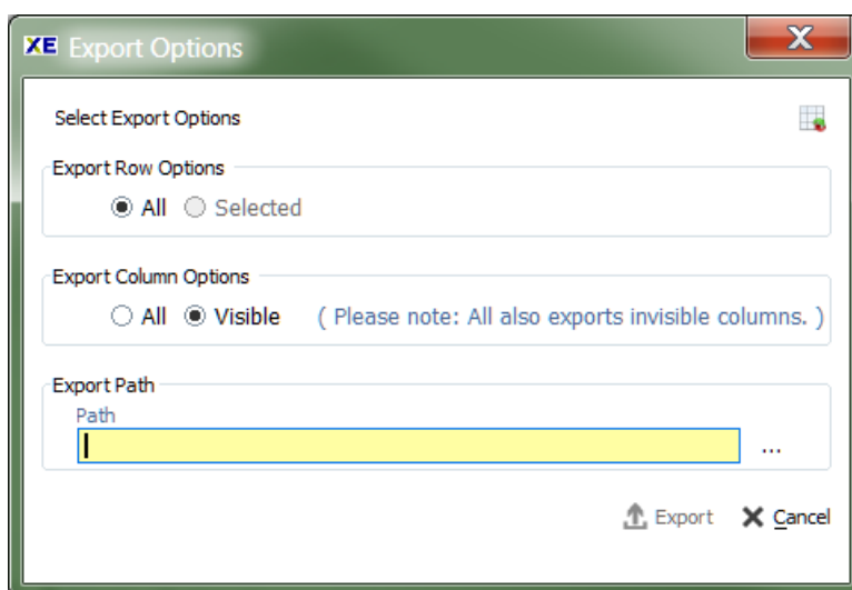
Fig. 30: Export Options
